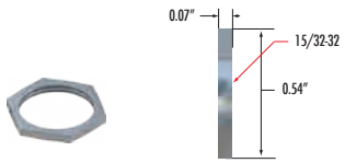
Hex Nut
